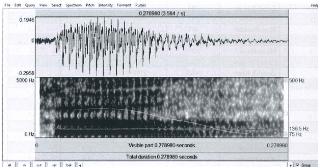
Слика 1. Осцилограм и сѣкѣрограм на консонанѣиш /ʍ/ (t) кај маѣки говориѣел
